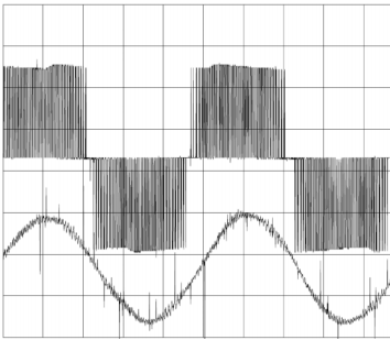
Umrichterausgangsspannung und -strom ohne Motor-Sinusfilter
