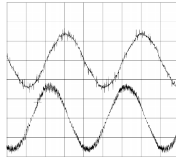
Umrichterausgangsspannung und -strom mit Motor-Sinusfilter
